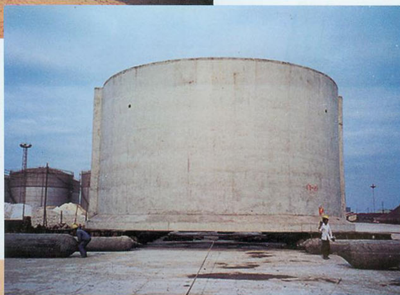
● 无底大圆筒采用气囊 加托板出运新工艺
